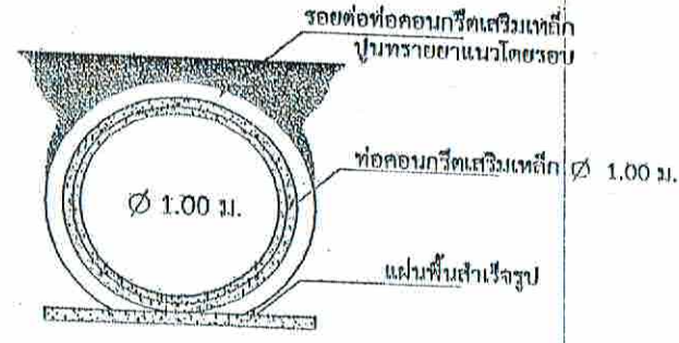
แบบขยาย B
